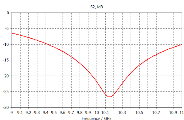
Потери в запертом режиме
