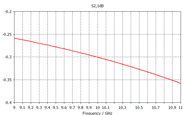
Потери в открытом режиме
